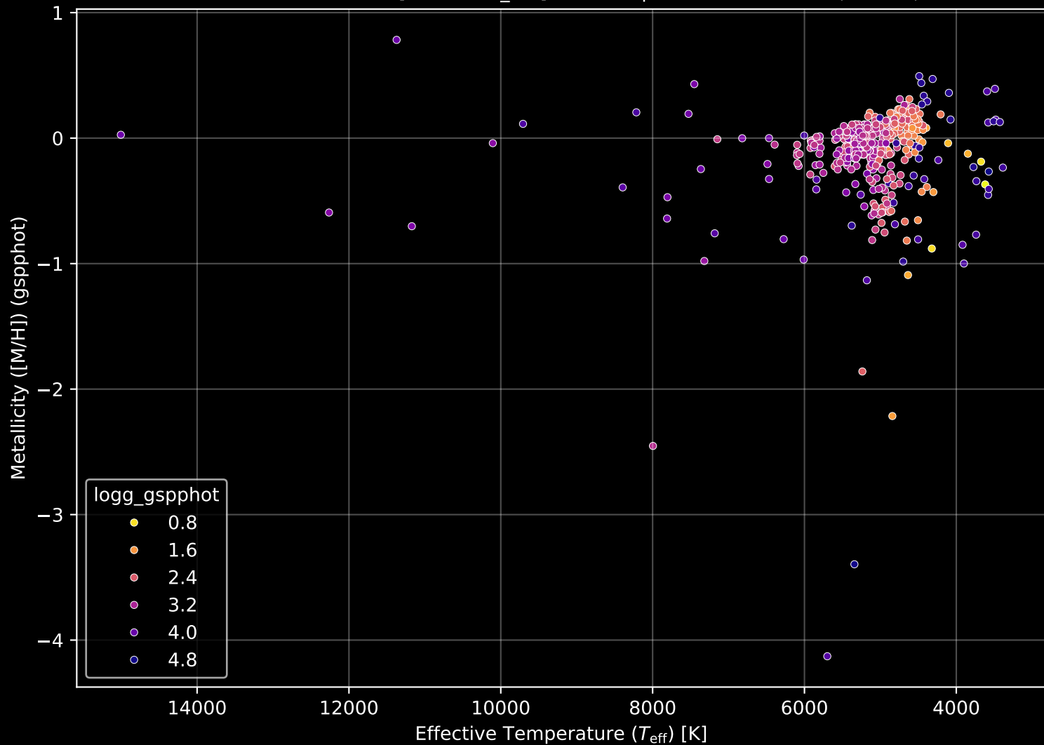
APOGEE DR17 Field: [TAUL1517_btx] Stellar Population Parameters (n= 470)
